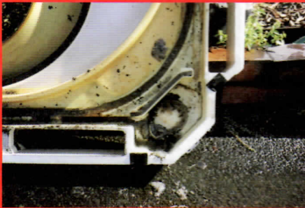
設置場所 飲食店舗 使用年数 4年 撮影面 ドレンパン 機種 4方向天井埋込型
