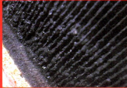
設置場所 飲食店舗 使用年数 5年 撮影面 熱交換面 機種 4方向天井埋込型
