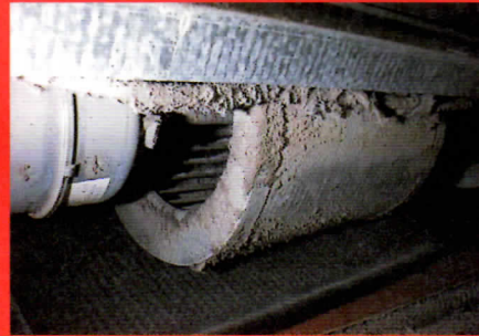
設置場所 医療機関待合室 使用年数 10年 撮影面 送風機 機種 床置き型
