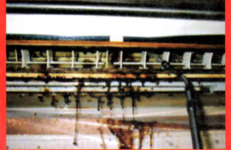
設置場所 守衛所 使用年数 3年 撮影面 吹き出し口 機種 壁掛け型
